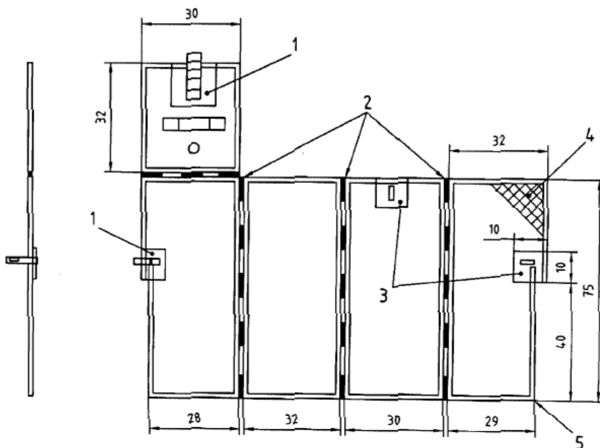
a) Bản vẽ chi tiết hộp thử
